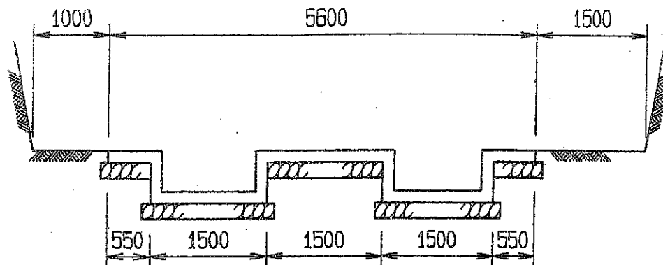
断面図
