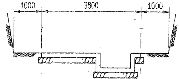
B-B 断面
