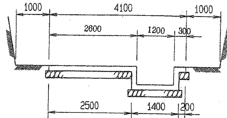
B-B 断面図
