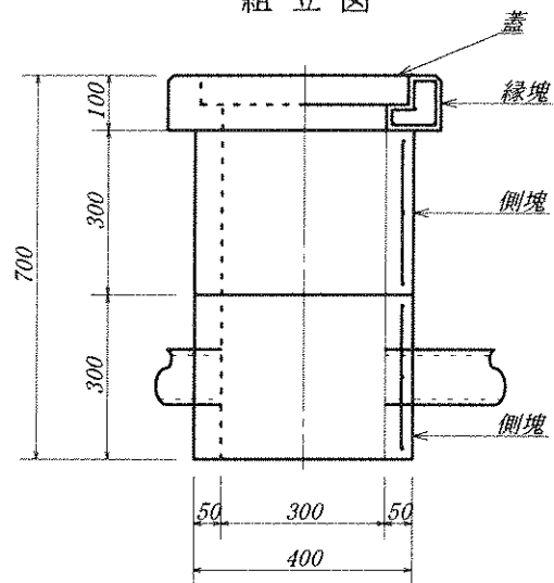
組立図
