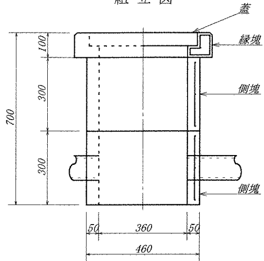
組立図
