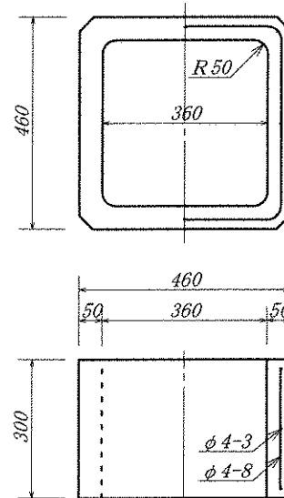
側塊
