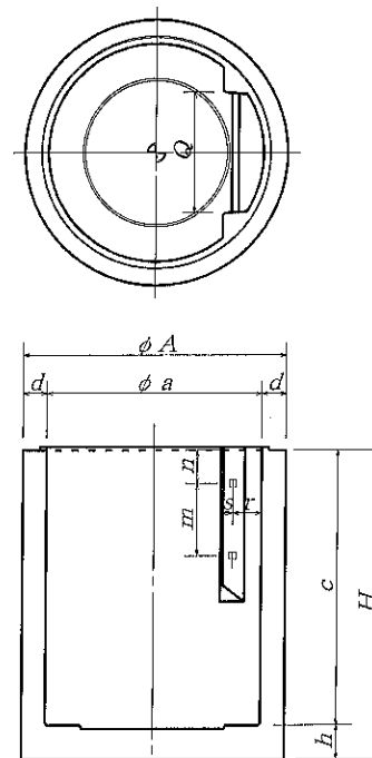
底板一体型管取付壁
