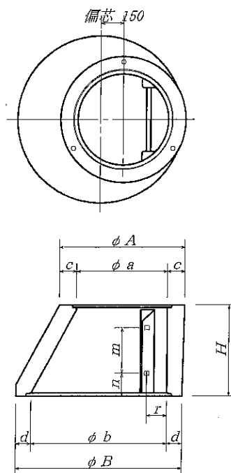
斜 壁
