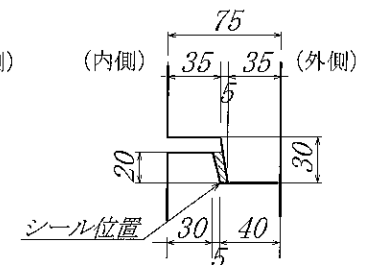
接合部詳細図
