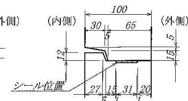
接合部詳細図
