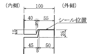
接合部詳細図
