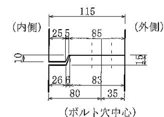
調整リング接合部詳細図
