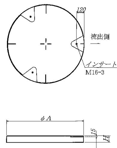
レベル底板
