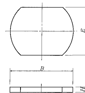
底 版
