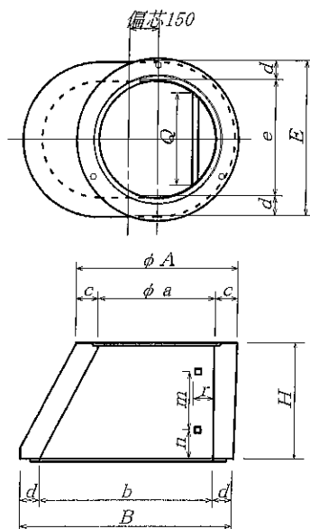
斜 壁
