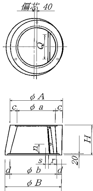
斜 壁
