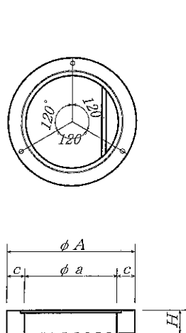
調整リング
