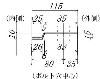
調整リング接合部詳細図
