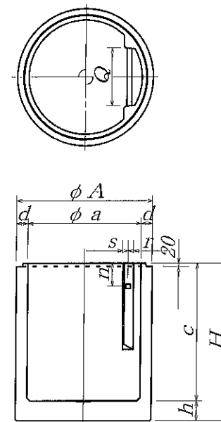
調整リング接合部詳細図
