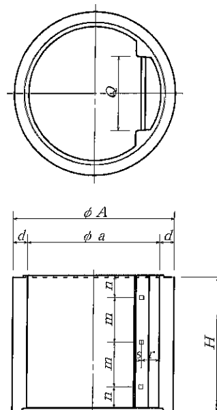
直 壁
